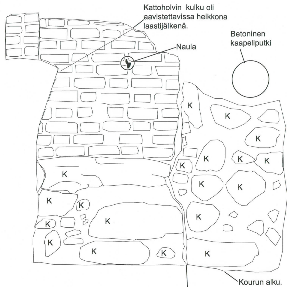
R114G SW-profilii (Päätysseinä)
