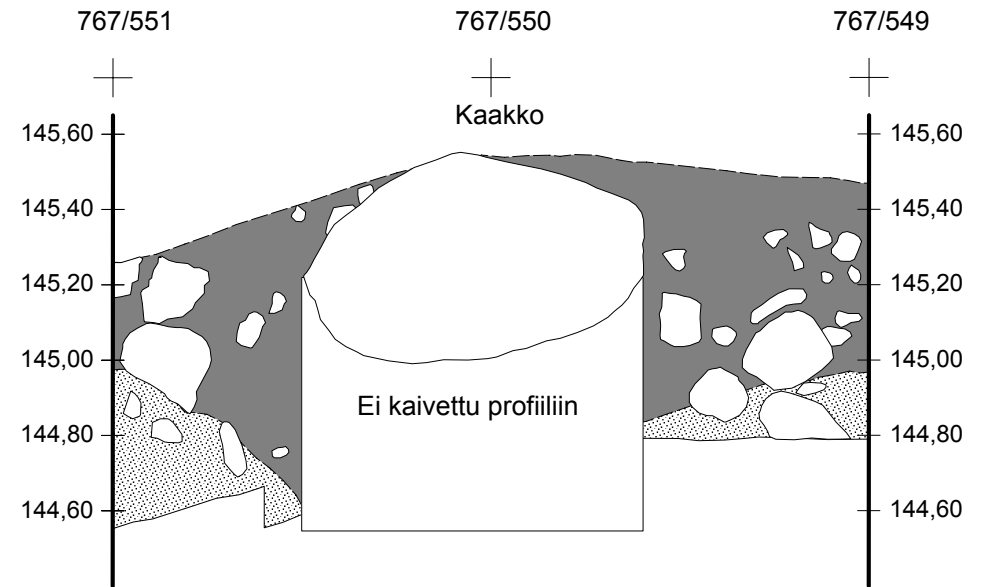
Kaakkoisprofiili
