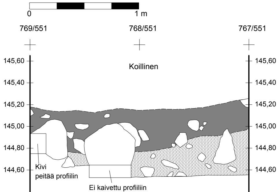
Koillisprofiili
