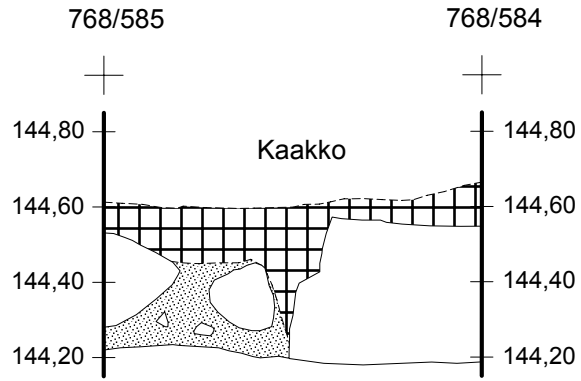
Kaakkoisprofiili
