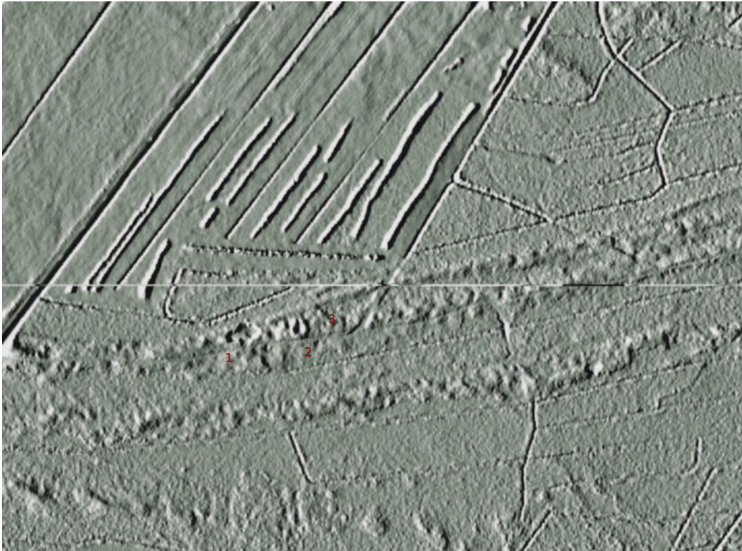
Kartta 4. Lidar-vinovalovarjoste. Muinaiset hiekkadyynit (kaarrot) erottuvat hyvin ympäristöstään. Lisäksi erottuu ihmisen aiheuttamia muutoksia: 1 sorakuoppa, 2 tervahauta, 3 tervapirtin pohja. Pitkäkaarto hankealueen lounaisosassa. Maanmittauslaitoksen Lidar pistepilviaineisto 05/2015.
