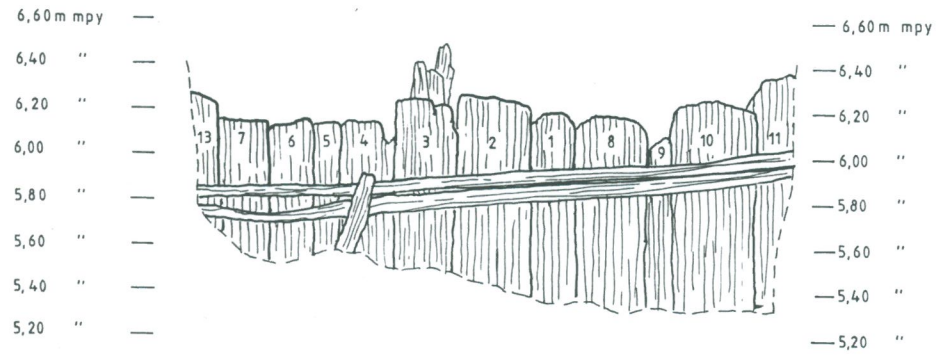
LEVITYSPIIRROS. (Tynnyrin seinä ulkopuolelta)
