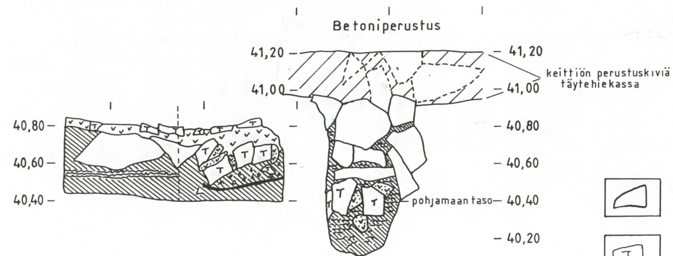
Tiilirakenne ja paalunsija, profiilit
