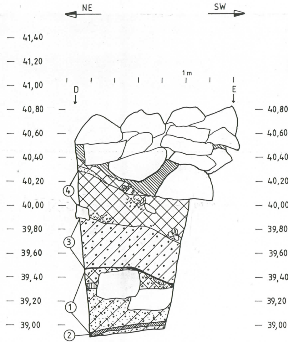
RA 2 b:n eteläprofiili
