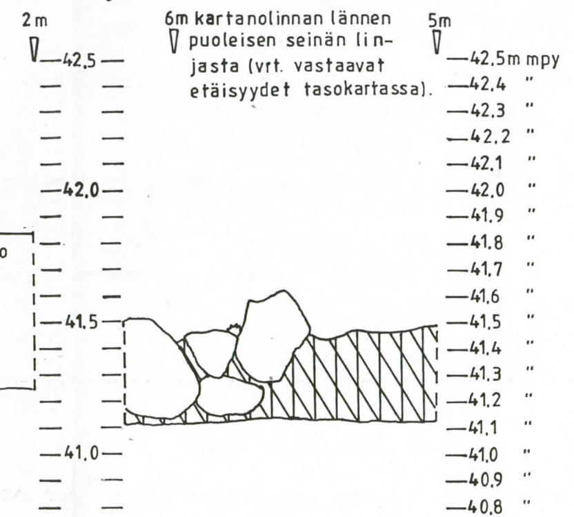
RA 6:n kiveyksen länsihaaran profiili pohjoisesta.
