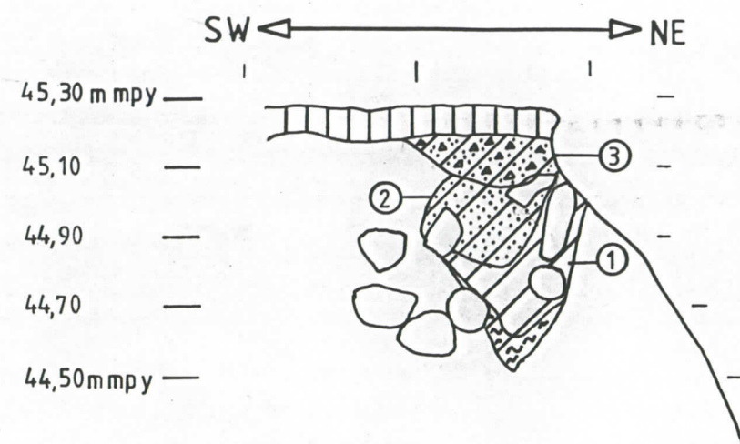
Y 3, KAIVANTO I, NW-PROFIILI
