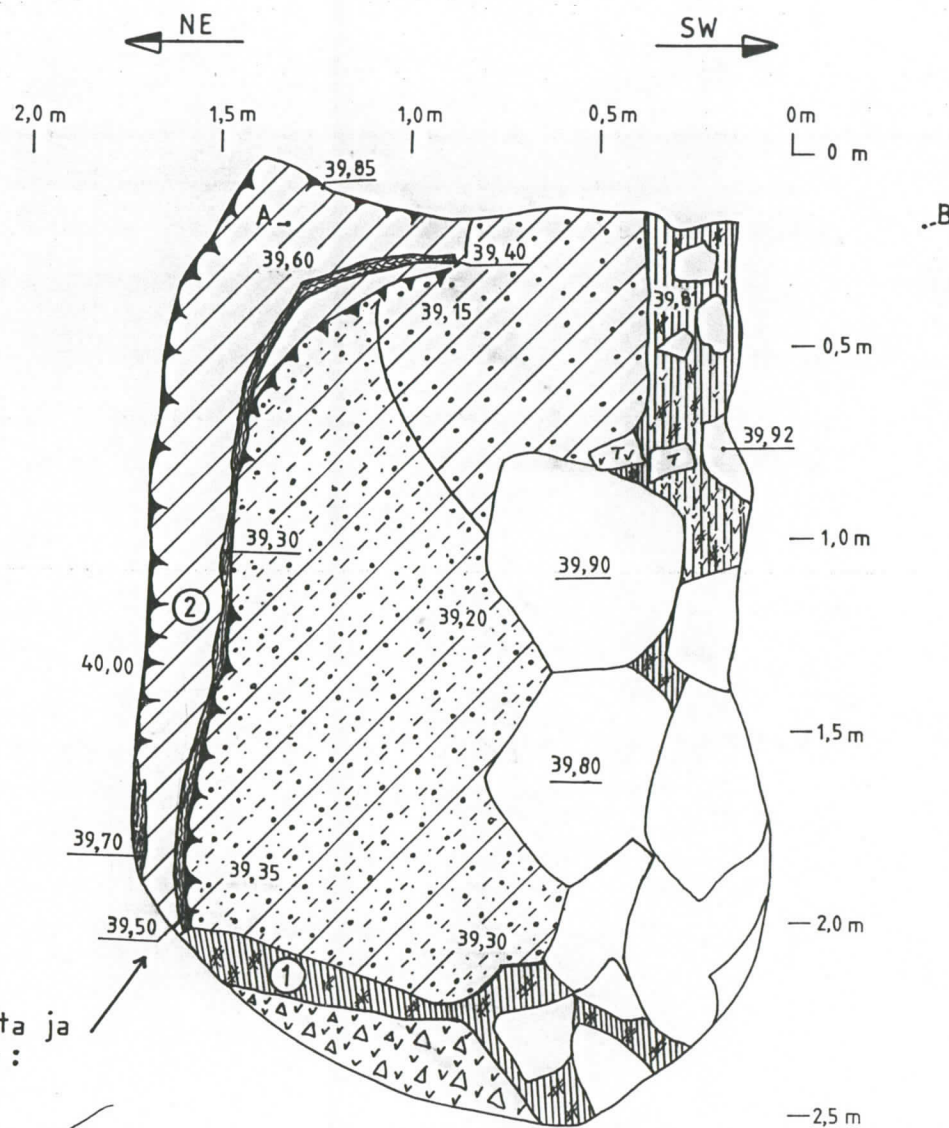
RA 2a, tasokartta
