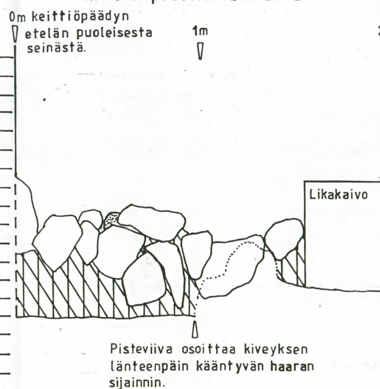
RA 6:n profiili lännestä.
