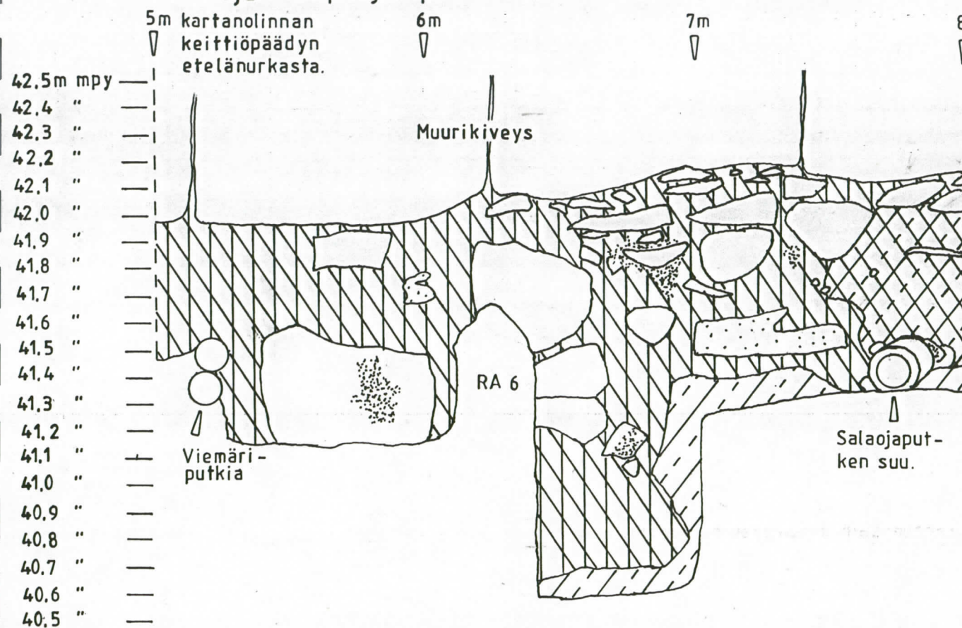
Ojan C3 pohjoisprofiili etelästä RA 6:n kohdalta.
