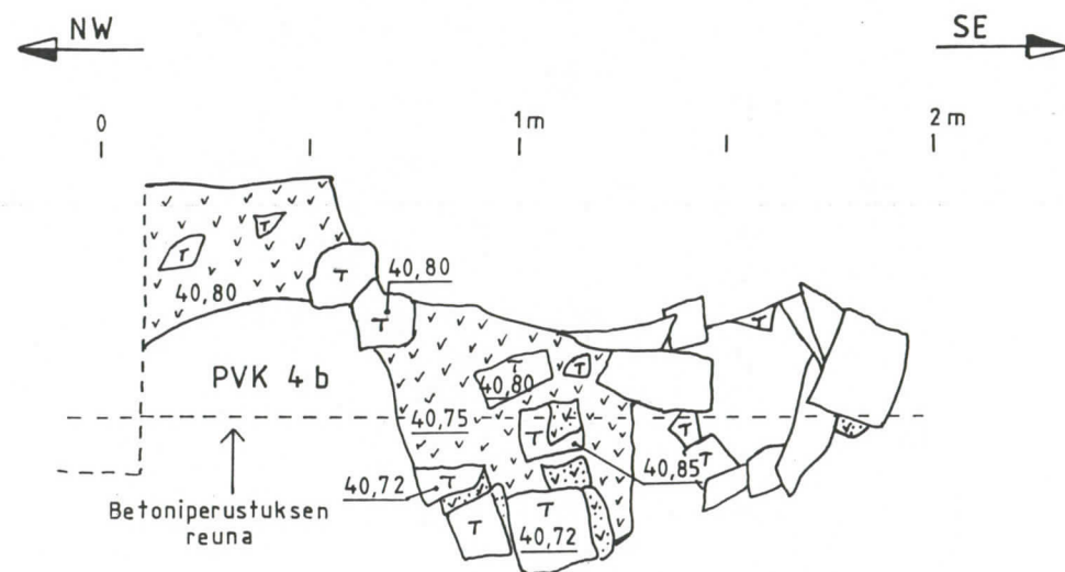
Tiilirakenne ja paalunsija, profiilit
