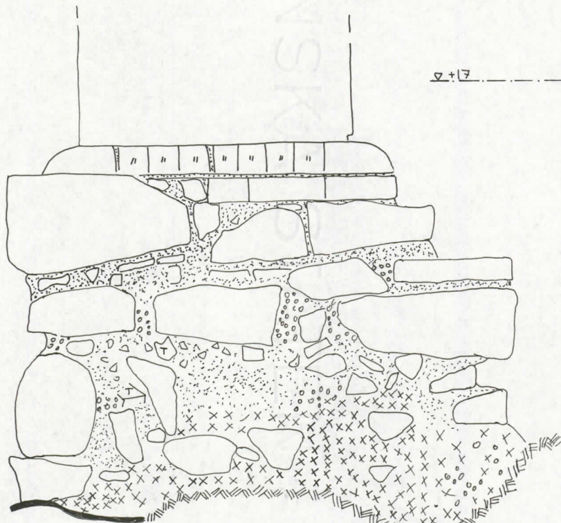
PILARI S 2 ITÄ 1:20
