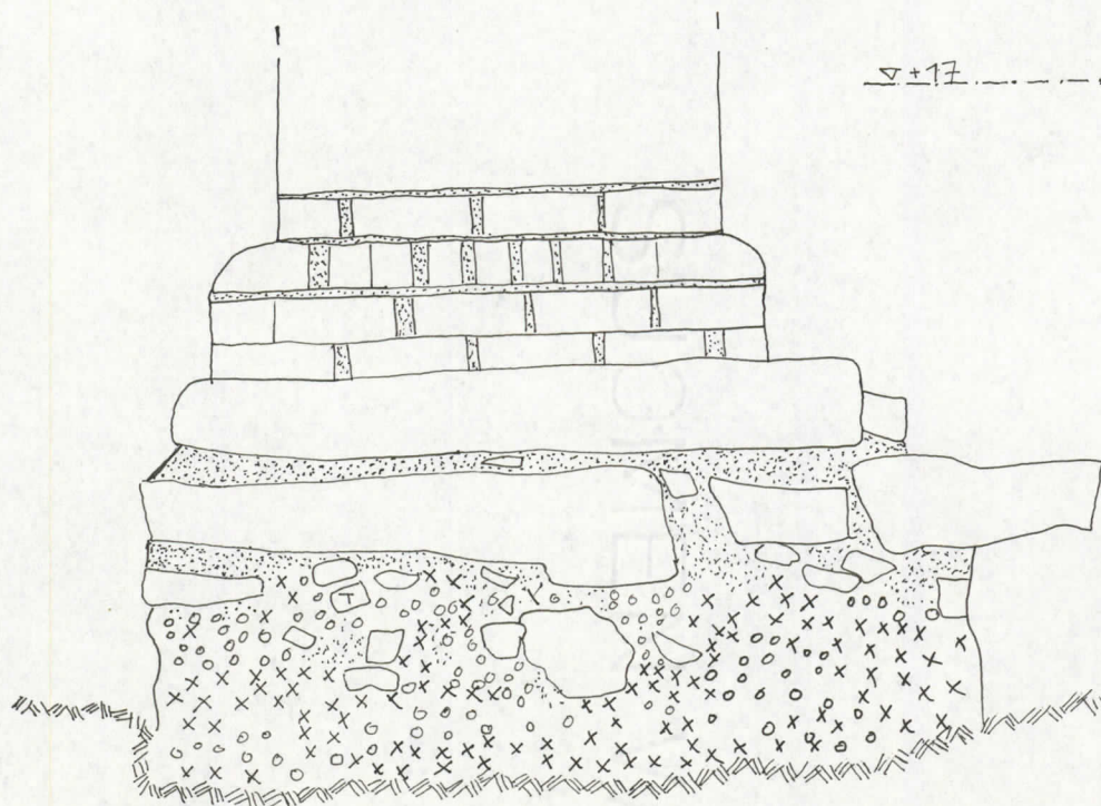
PILARI N 3 ITÄ 1:10
