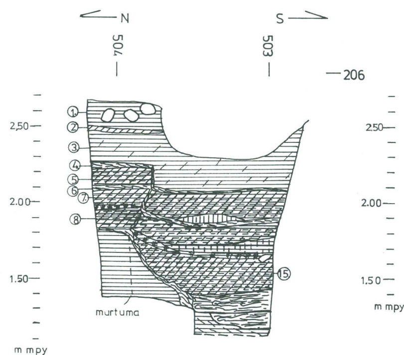
Itäprofiili 1:25 (b-b)
