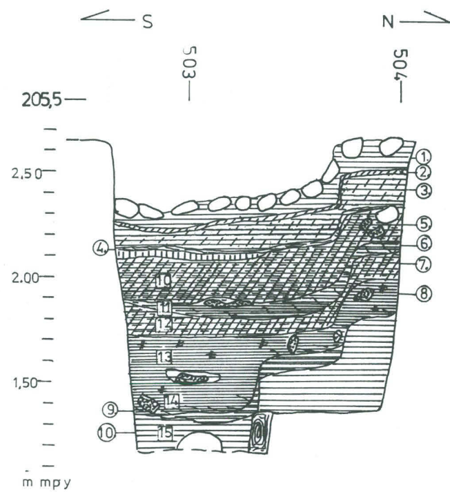
Länsiprofiili 1:25 (a-a)
