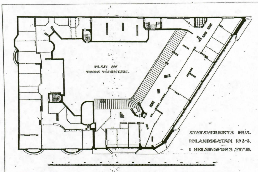
Kiinteistön Uudenmaank. 1-3-5 ullakkokerros joulukuussa 1916. Mittausspiirustus, YRYH, P. af Enehjelm ja R. Finnilä. VA Rakh II.
