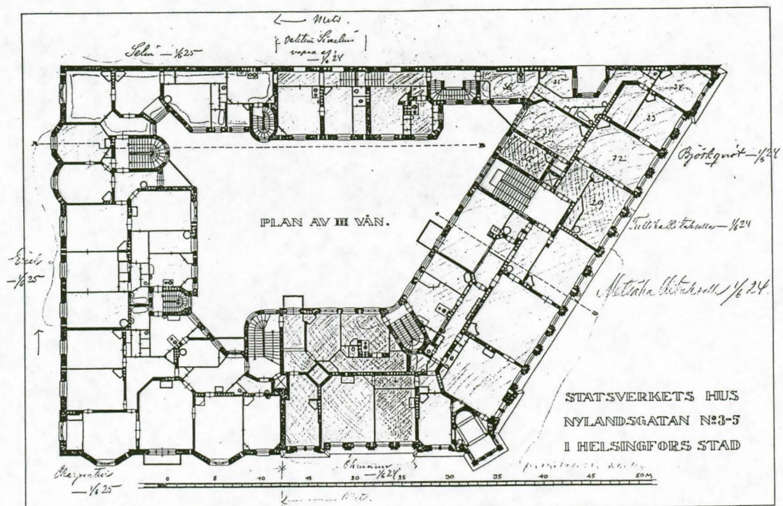
Kiinteistön Uudenmaank. 1-3-5 toinen ja kolmas kerros joulukuussa 1916. Mittauspöyrustukset, YRYH, P. af Enehjelm ja R. Finnilä. VA Rakh II.
