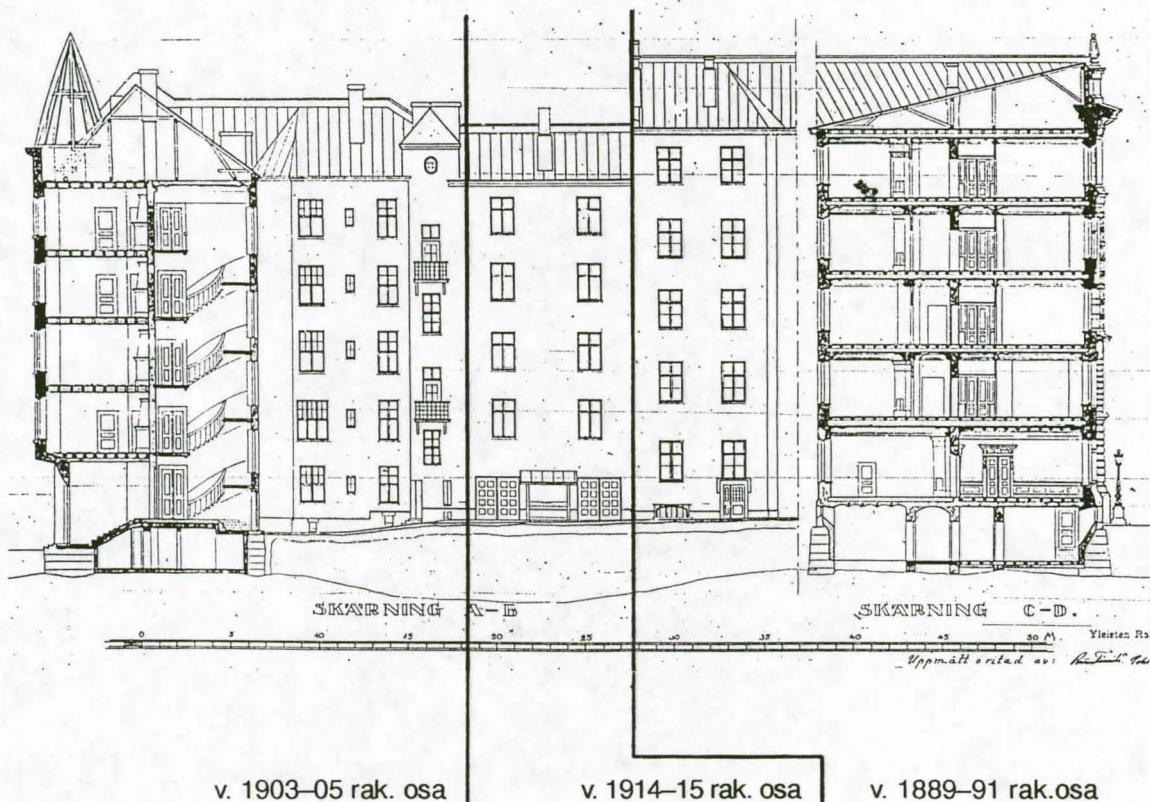
Kiinteistö Uudenmaankatu 1–3–5 joulukuussa 1916. Mittauspiirustus, YRYH, P. af Enehjelm ja R. Finnä. VA Rakh II.
