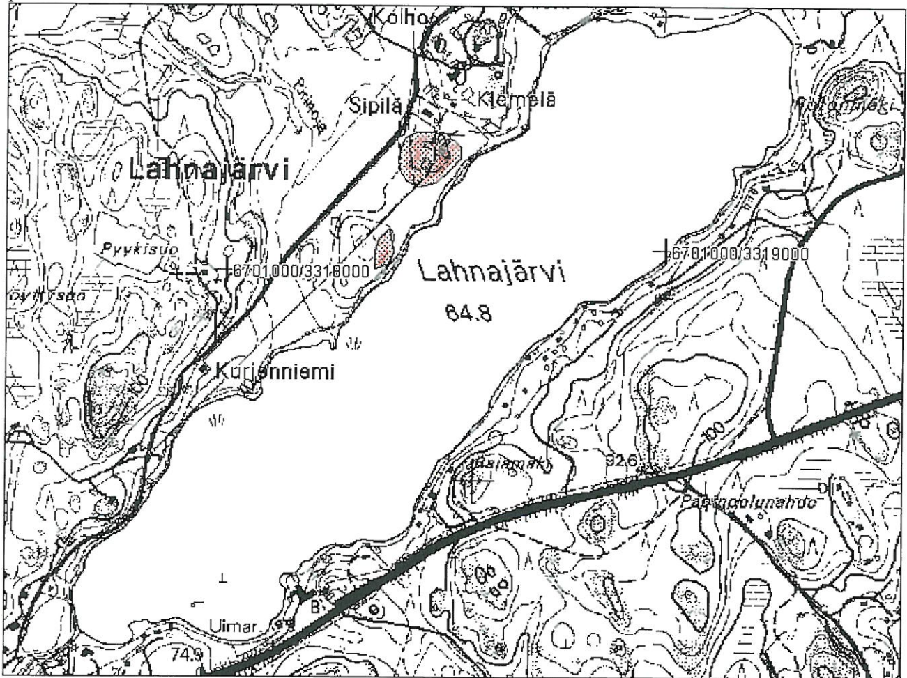
Ote peruskartasta 20213 08 Lahnajärvi (1:20 000)
