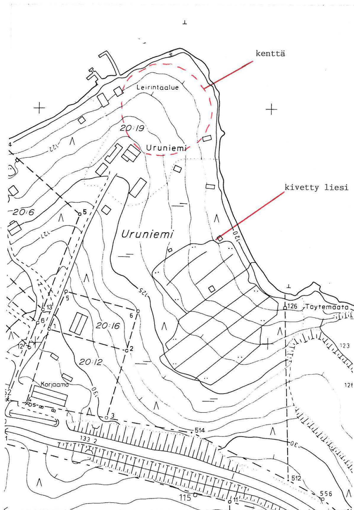
Ote kaavoituksen pohjakartasta 1:2000
