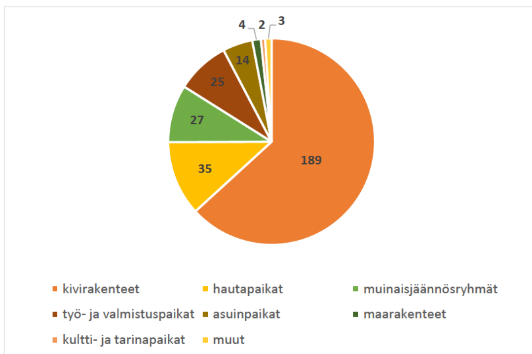
Kuva 7. Laihian kiinteiden muinajäännöskohteiden (n=299) jakautuminen tyypeittäin SKAIK-projektin inventointien jälkeen. Yksittäisissä kohteissa voi olla useita kymmeniä erillisiä rakenteita eli alakohteita, kuten kivilatomuksia, asumuspainanteita tai keitto-kuoppia.
