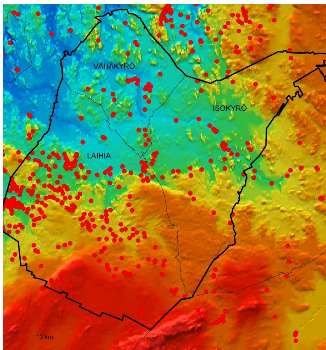
Kuva 3. Korkeusmalli Kyrönmaan seutukunnasta ympäristöineen. Kivikautisia rannankorkeuksia on korostettu kartalle punaisella, pronssikautisia keltaisella ja rautakautisia vihreällä värillä. Punaiset pallot kuvaavat muinaisjäännösrekisterin kohteita. Korkeusaineisto MML, muinaisjäännösrekisteriaineisto Museovirasto. Visualisointi: Satu Koivisto/SAIK.
